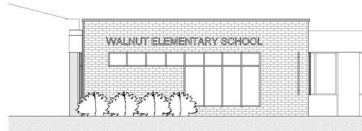
WEST ELEVATION SCALE: 3/8" = 1'-0"
